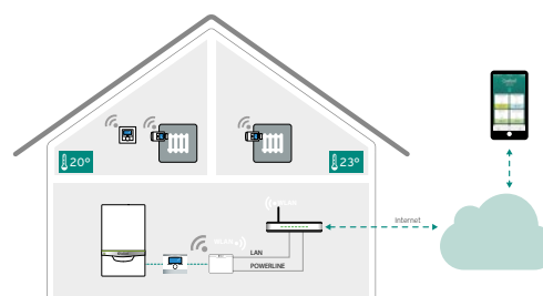
Schemat działania systemu regulacji temperatury ambiSENSE
