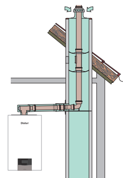
Przyłącze do przewodu spalinowego \varnothing 80 mm (w szachcie)
